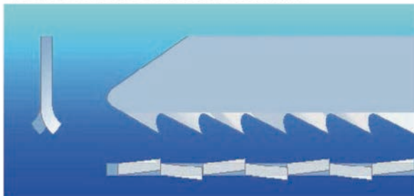
Dientes Fresados corte libre Triscado
